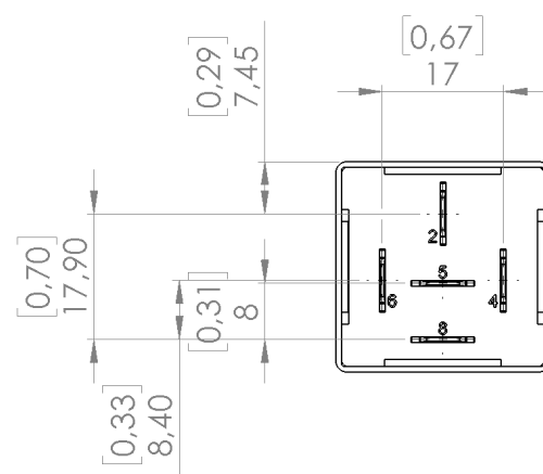
Ansicht von unten, Typ S1/S3
