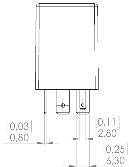
Seitenansicht Typ S2
