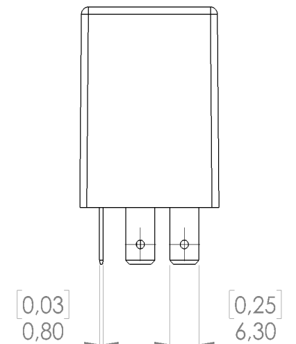
Seitenansicht Typ S1/S3
