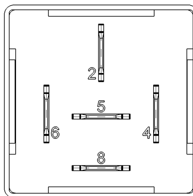
Pingelegung S1/S3 , Ansicht von unten
