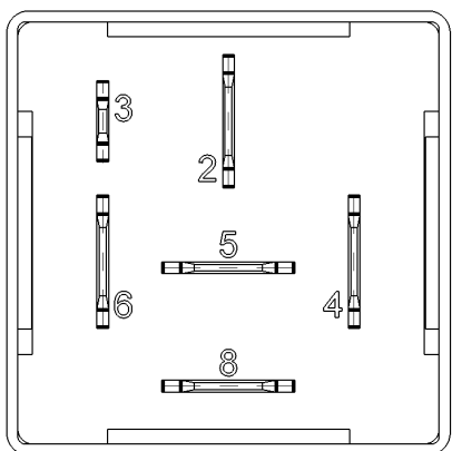
Pingelegung S2 , Ansicht von unten
