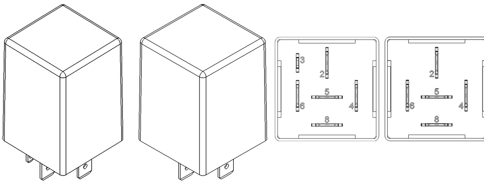
Einbauansicht S2
