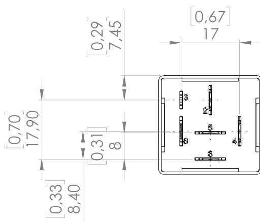
Ansicht von unten, Typ S2
