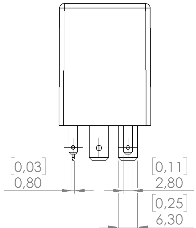
Seitenansicht
