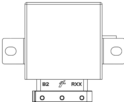
Einbauansicht
