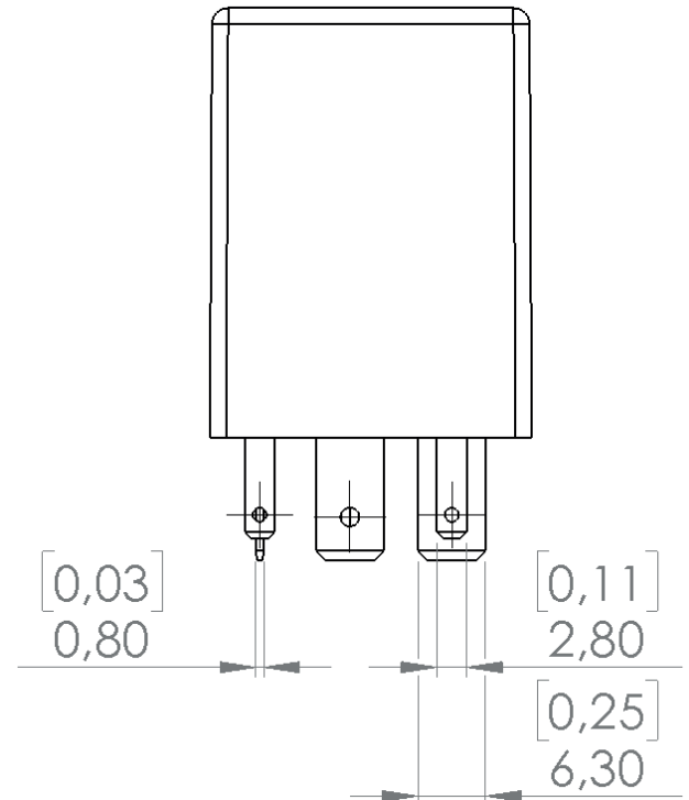
Seitenansicht
